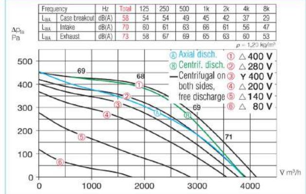
GBD 400/4/4 T120
